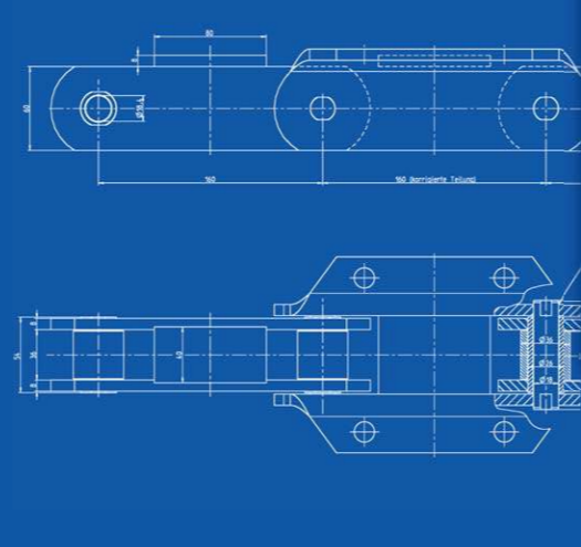
Becherwerkskette
